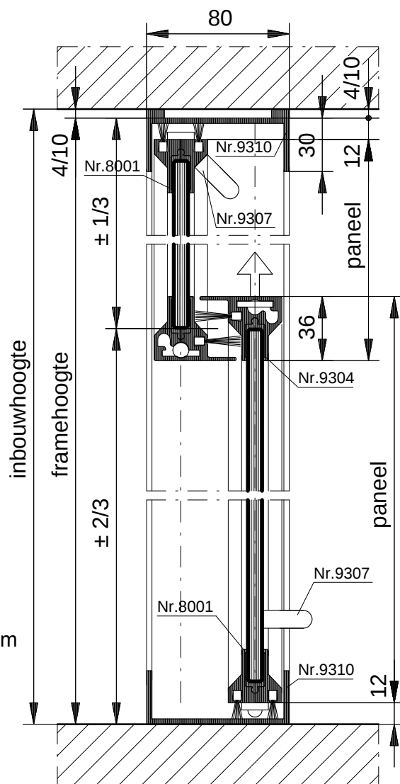
VERTICALE DOORSNEDE type VSV-3
