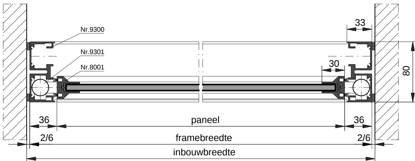
HORIZONTALE DOORSNEDE type VSV-3
