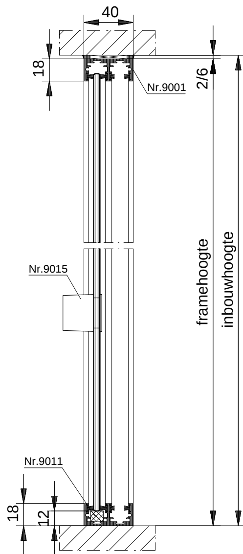
VERTICALE DOORSNEDE type HSV-3
