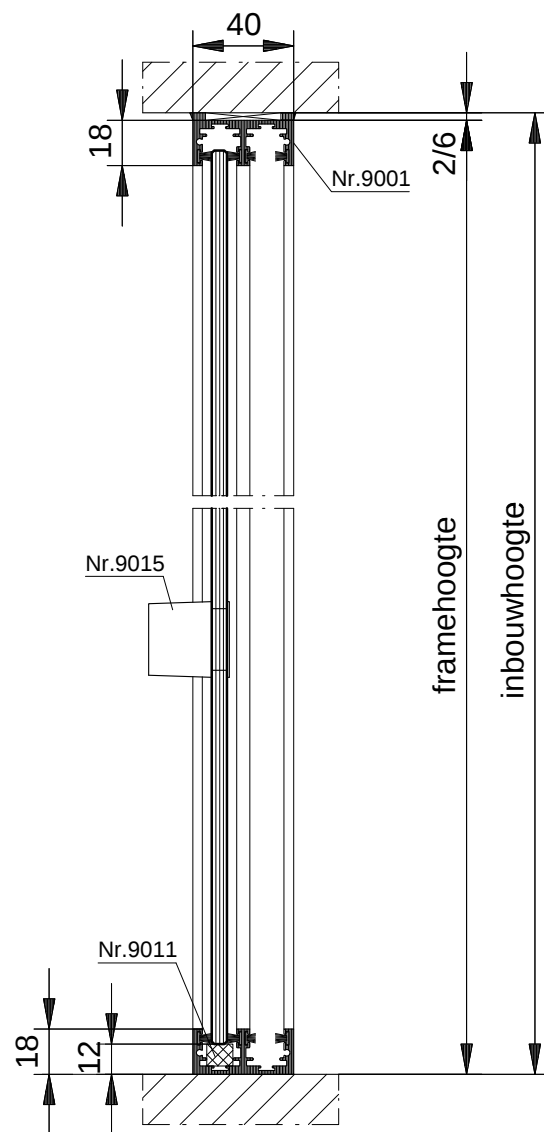
VERTICALE DOORSNEDE type HSV-2
