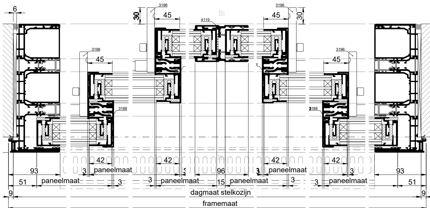
HORIZONTALE DOORSNEDE type XHS-9E
