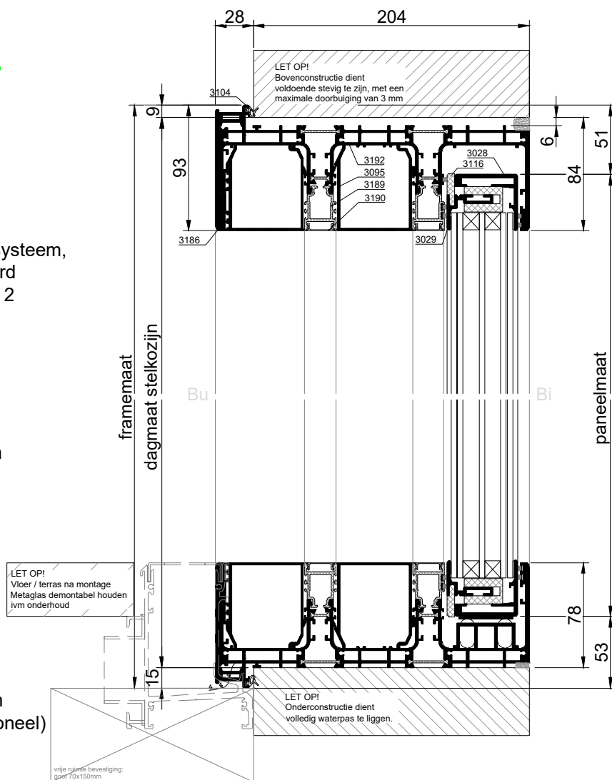
VERTICALE DOORSNEDE type XHS-9A
