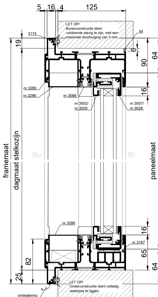
VERTICALE DOORSNEDE type XHS-17C
