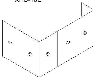
hoekopstelling vast glas XHS-9/10
