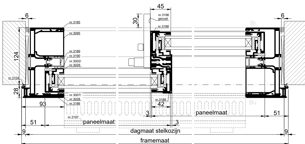
HORIZONTALE DOORSNEDE type XHS-9A
