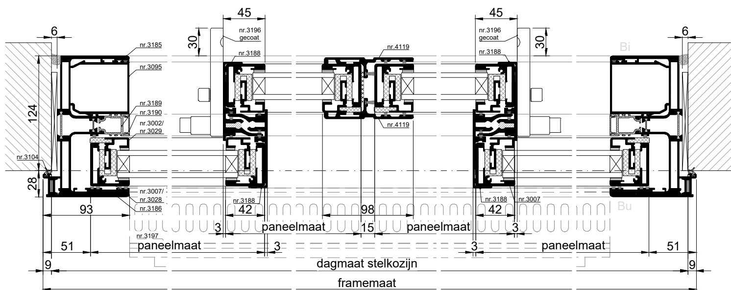
HORIZONTALE DOORSNEDE type XHS-9E
