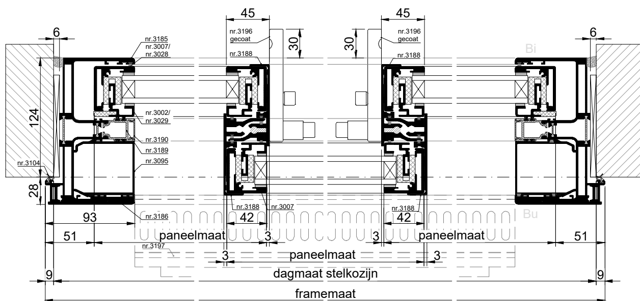
HORIZONTALE DOORSNEDE type XHS-9D
