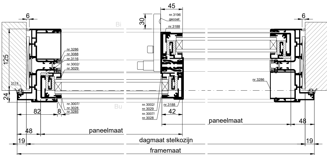
HORIZONTALE DOORSNEDE type XHS-17A
