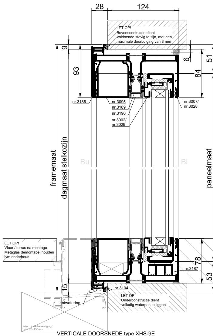
VERTICALE DOORSNEDE type XHS-9E
