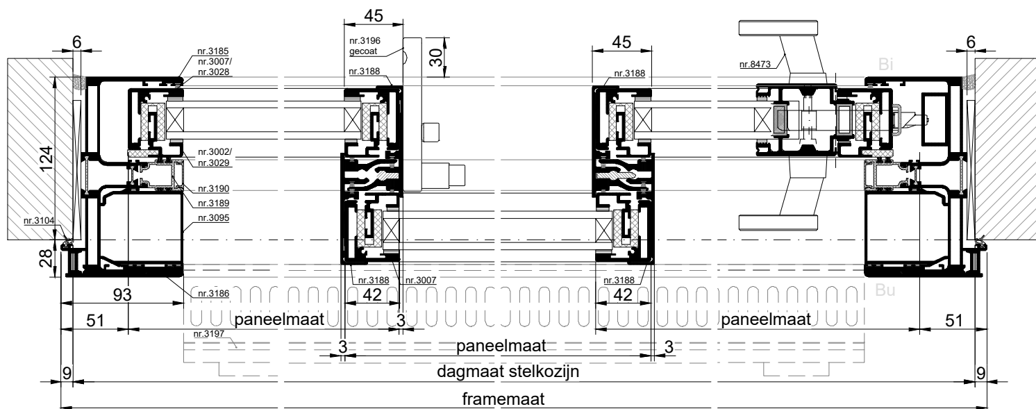
HORIZONTALE DOORSNEDE type XHS-10D
