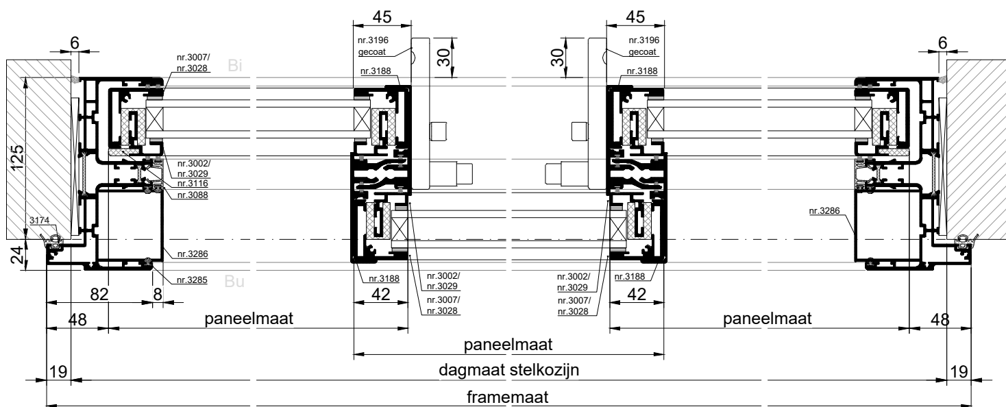
HORIZONTALE DOORSNEDE type XHS-17D
