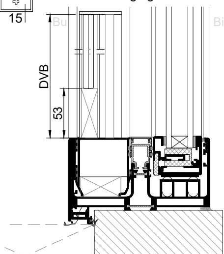
horizontaal onderprofiel met doorvalbeveiliging
