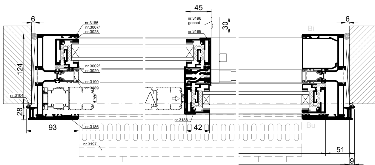
HORIZONTALE DOORSNEDE type XHS-9A
