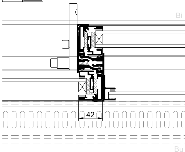
verticale middennaad met doorvalbeveiliging
