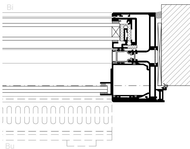
horizontaal onderprofiel met doorvalbeveiliging
