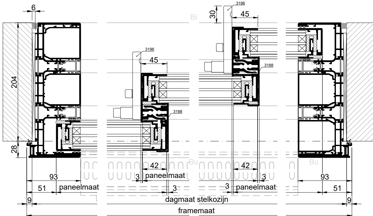
HORIZONTALE DOORSNEDE type XHS-9A
