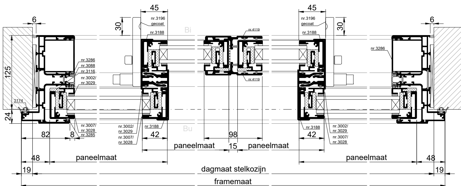
HORIZONTALE DOORSNEDE type XHS-17E
