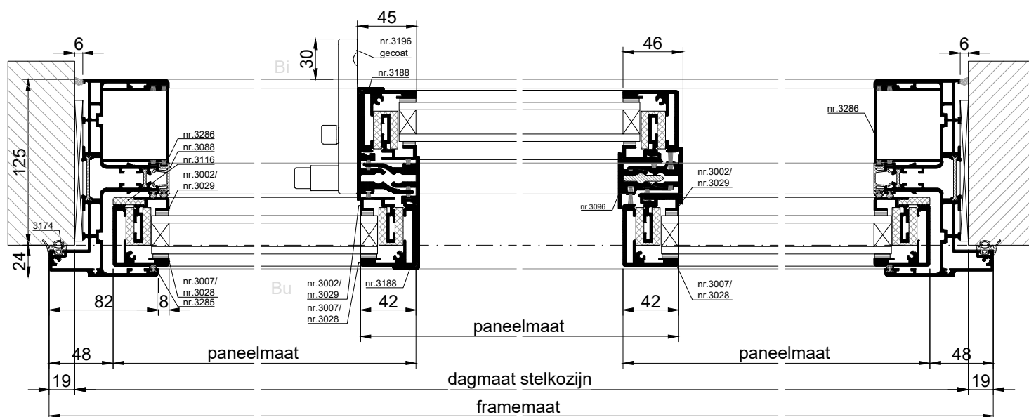
HORIZONTALE DOORSNEDE type XHS-17C
