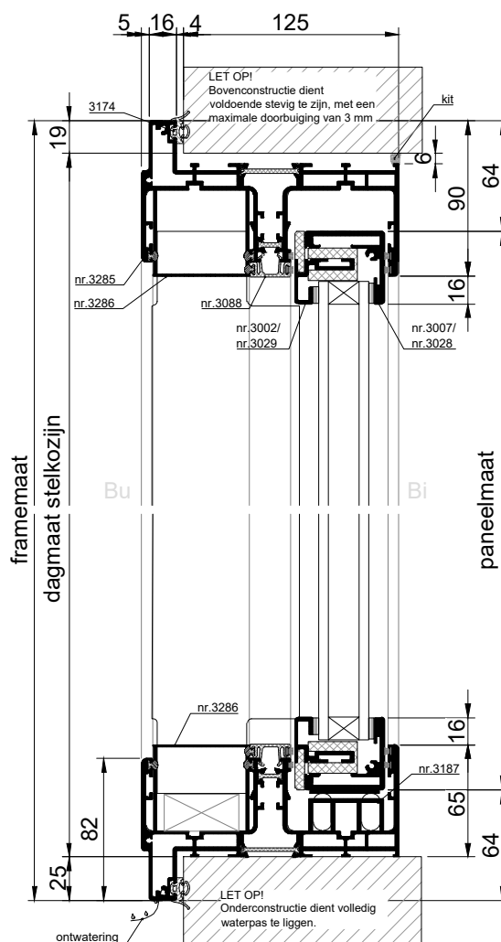
VERTICALE DOORSNEDE type XHS-17E
