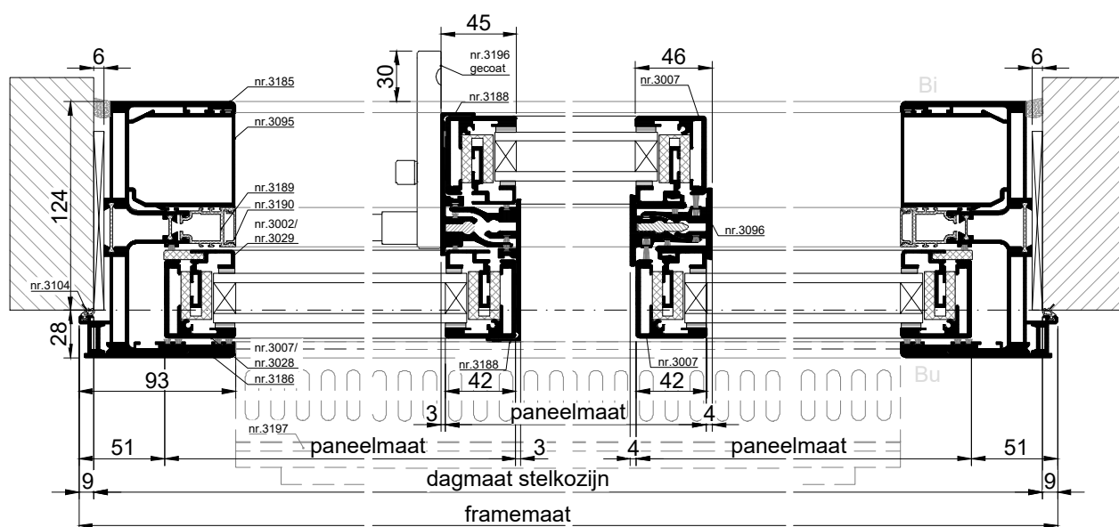
HORIZONTALE DOORSNEDE type XHS-9C
