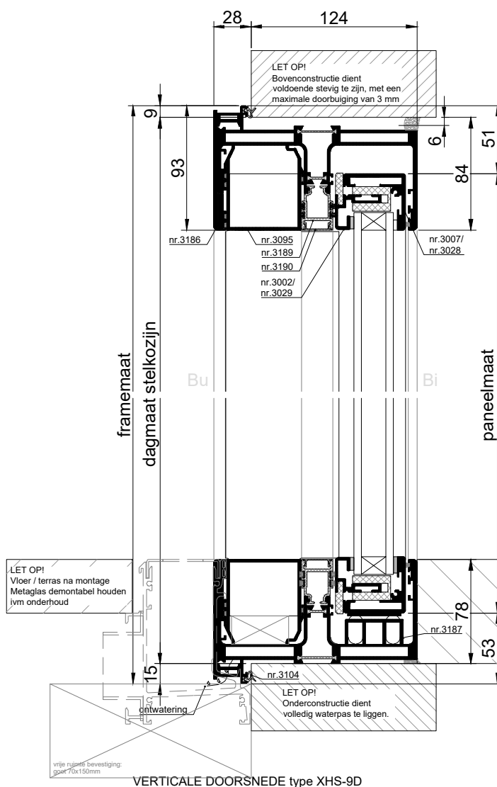
VERTECALE DOORSNEDE type XHS-9D
