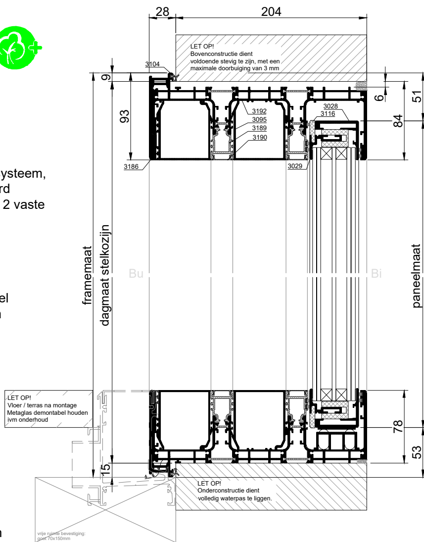
VERTICALE DOORSNEDE type XHS-9E
