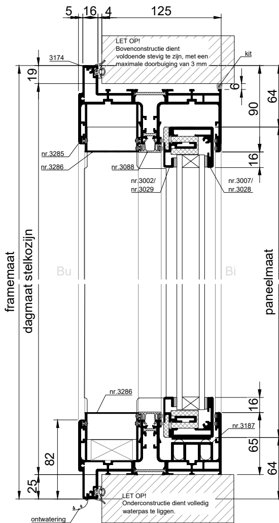
VERTICALE DOORSNEDE type XHS-17A
