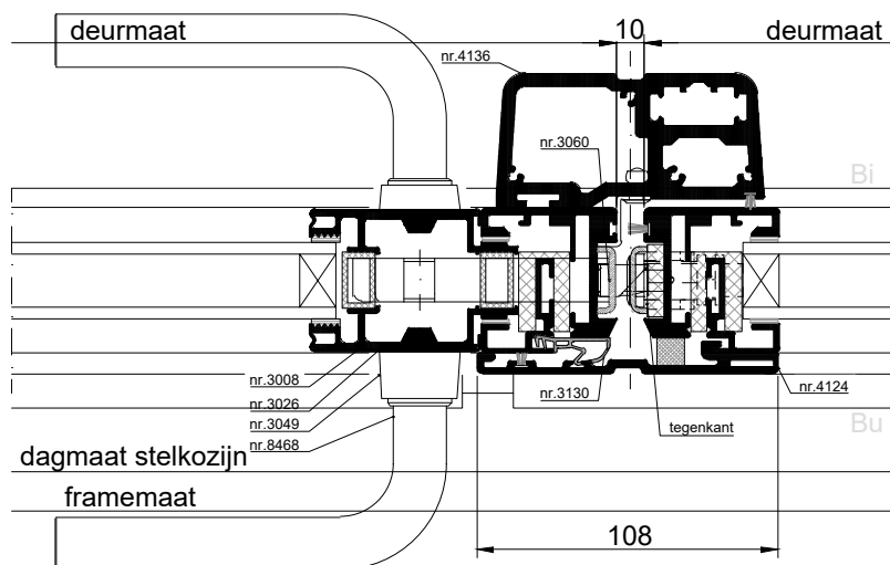
HORIZONTALE DOORSNEDE type XIS-1A/E
