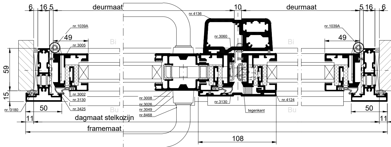
HORIZONTALE DOORSNEDE type XIS-1A
