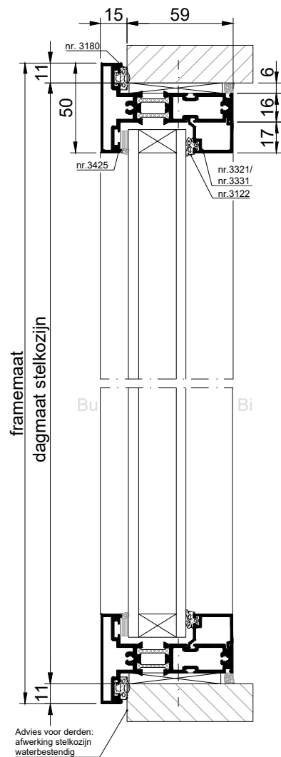
VERTICALE DOORSNEDE type XVI-1
