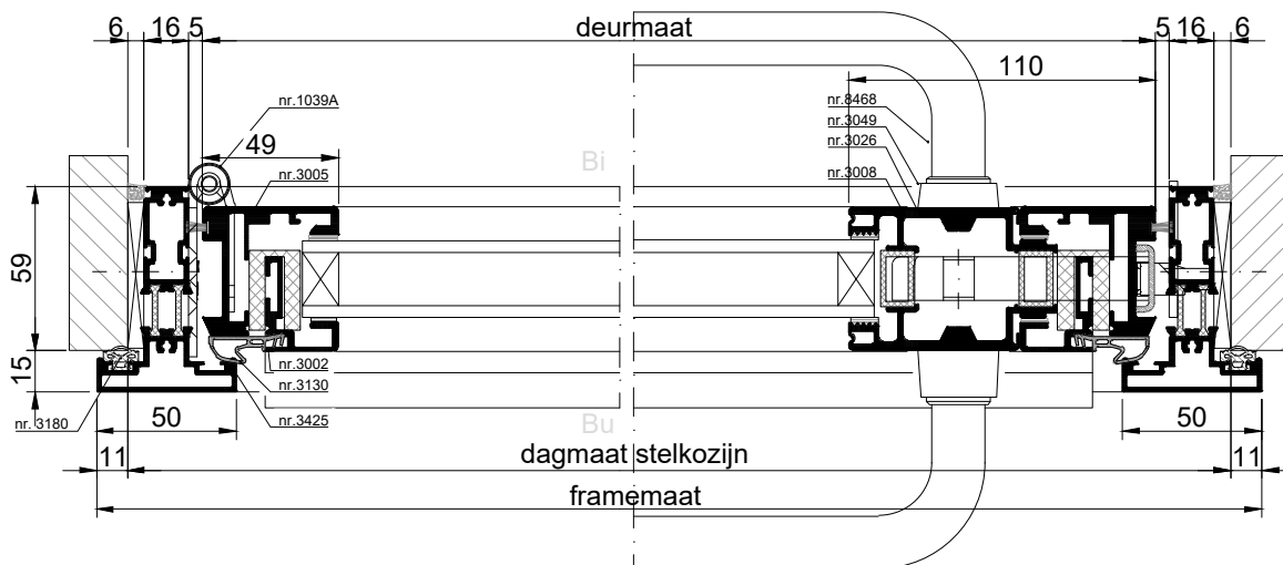
HORIZONTALE DOORSNEDE type XID-1A
