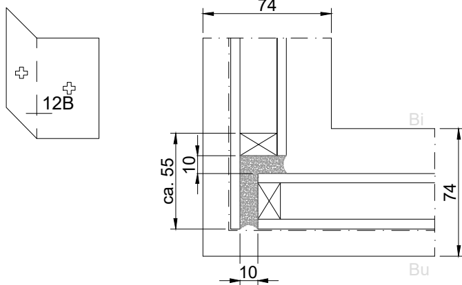
structurele glasverbinding zonder afdekprofiel
