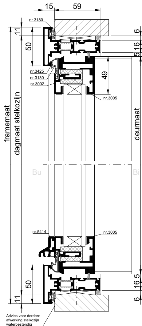
VERTICALE DOORSNEDE type XIS-1A
