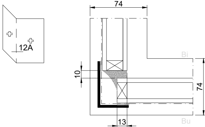
structurele glasverbinding incl. afdekprofiel
