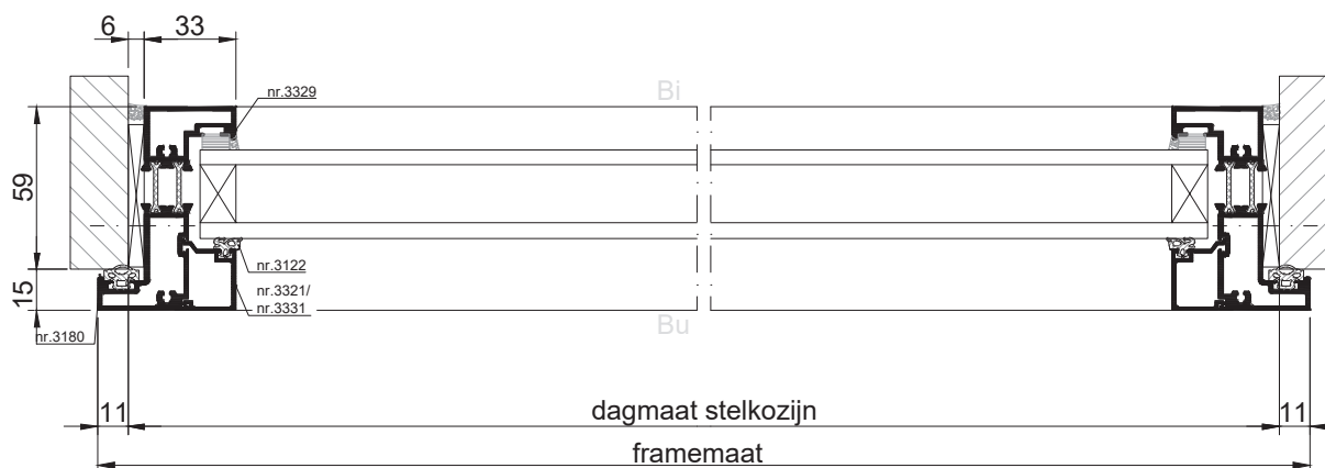
HORizontale DOORSNEDE type XVU-1
