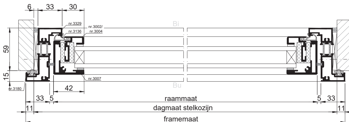
HORizontale DOORSNEDE type XKR-1
