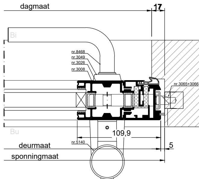
HORIZONTALE DOORSNEDE type MUD-6G/H
