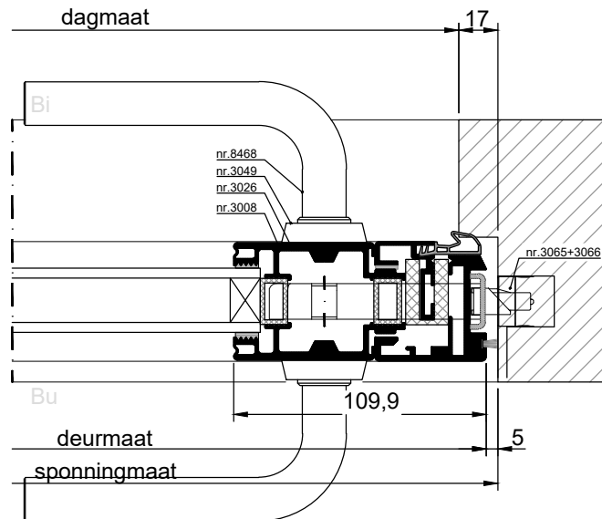
HORIZONTALE DOORSNEDE type MUD-6A/E
