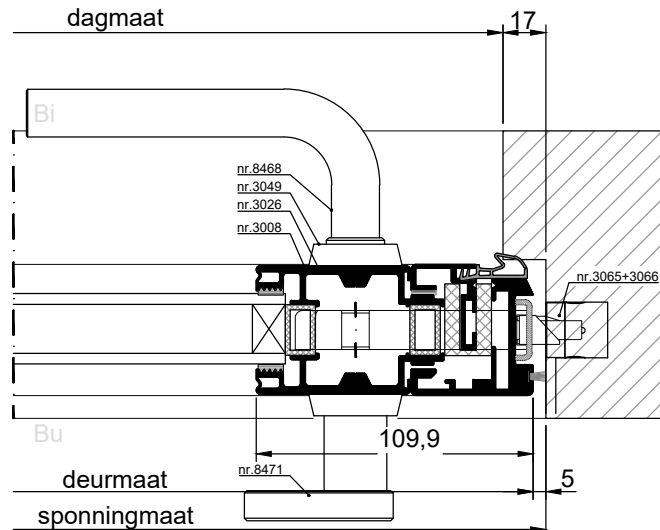
HORIZONTALE DOORSNEDE type MUD-6B/C/D/F
