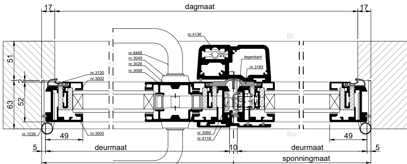
HORIZONTALE DOORSNEDE type MUS-6A
