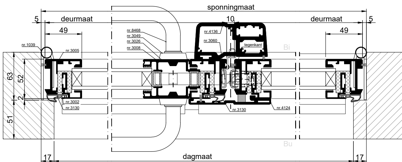
HORIZONTAL DOORSNEDE type MIS-6A
