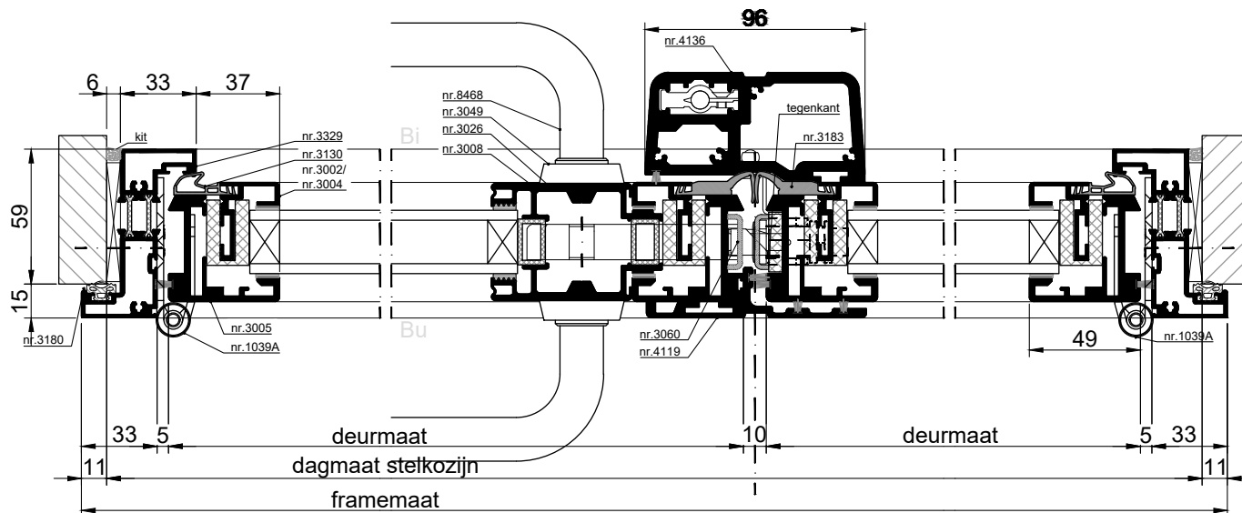
HORIZONTALE DOORSNEDE type XUS-1A
