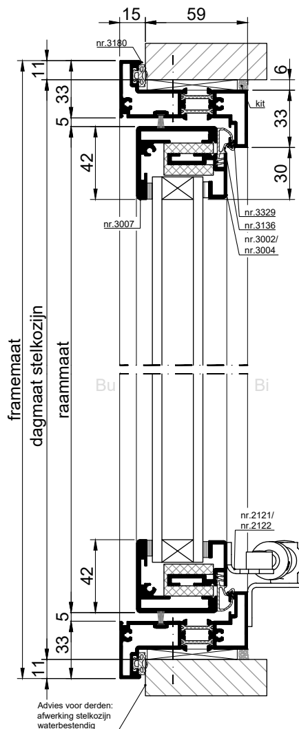
VERTICALE DOORSNEDE type XDU-1A
