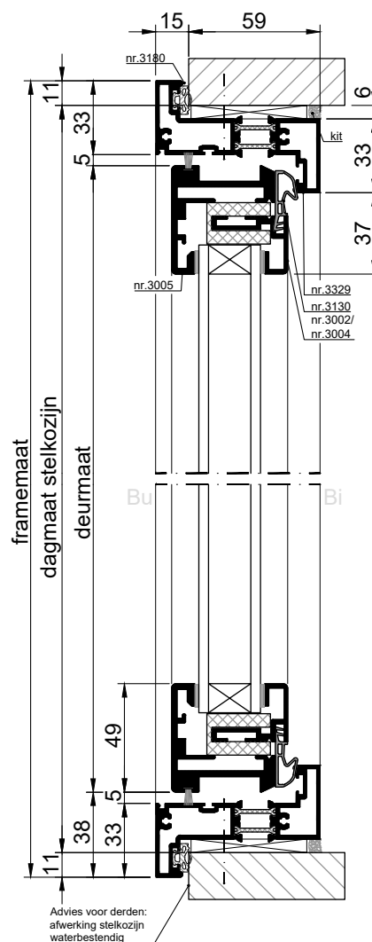
VERTICALE DOORSNEDE type XUD-1A
