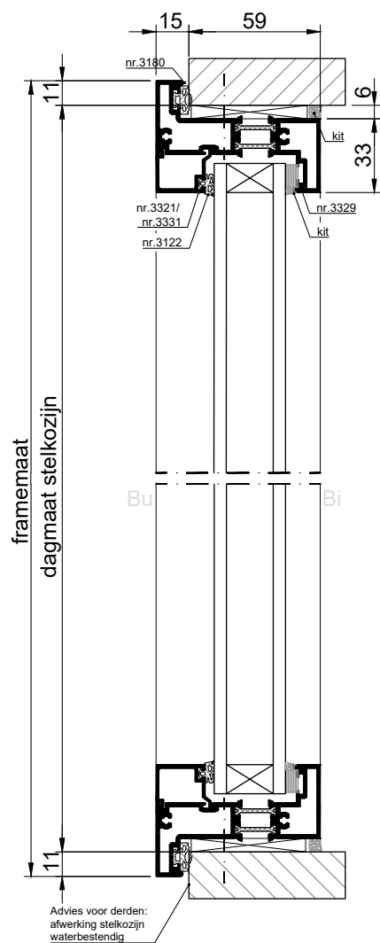
VERTICALE DOORSNEDE type XVU-1
