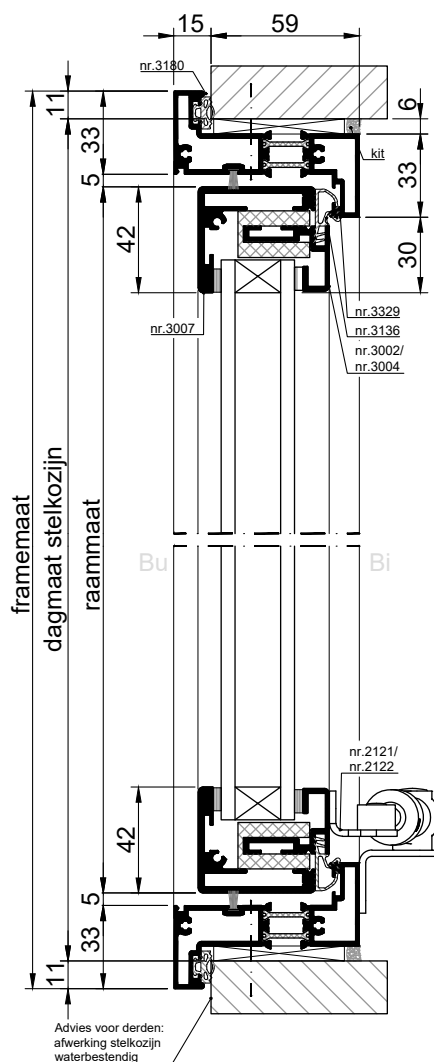
VERTICALE DOORSNEDE type XDU-1B
