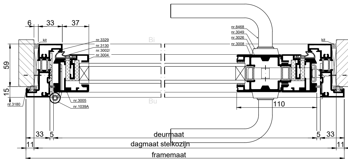
HORizontale DOORSNEDE type XUD-1A
