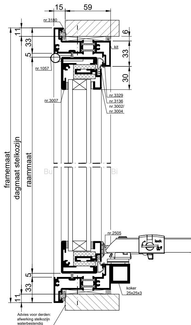
VERTICALE DOORSNEDE type XKR-1
