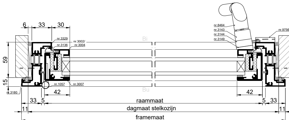
HORIZONTALE DOORSNEDE type XDU-1A
