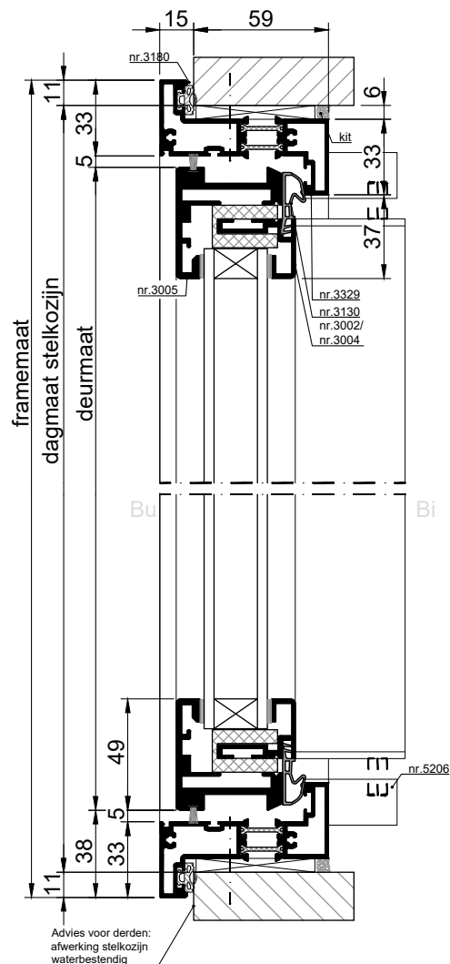
VERTICALE DOORSNEDE type XUS-1A
