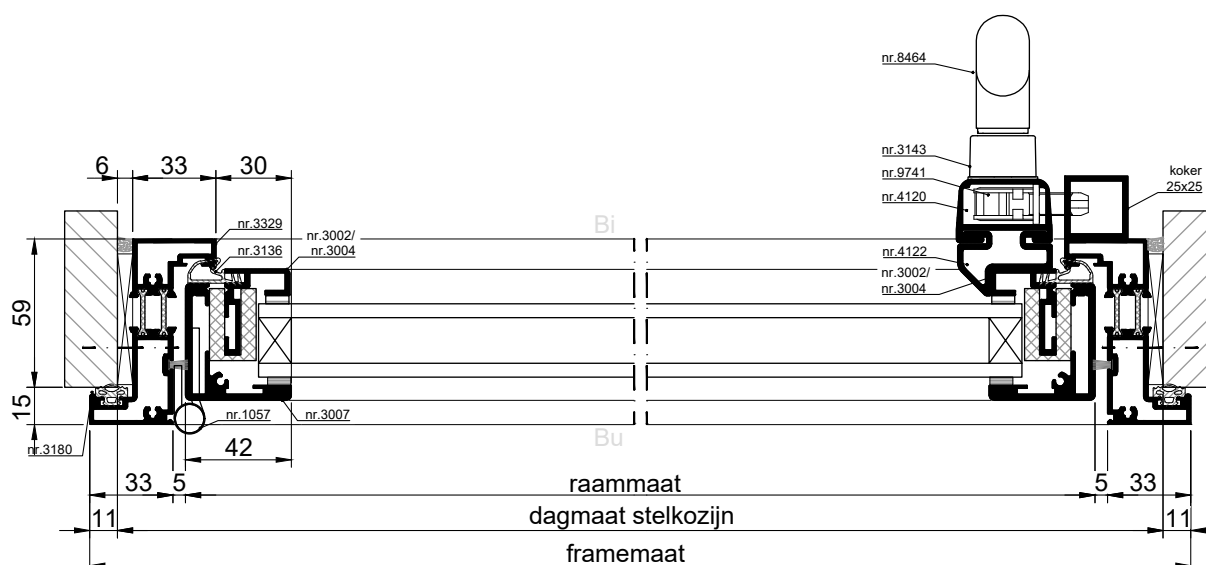
HORIZONTALE DOORSNEDE type XDU-1B
