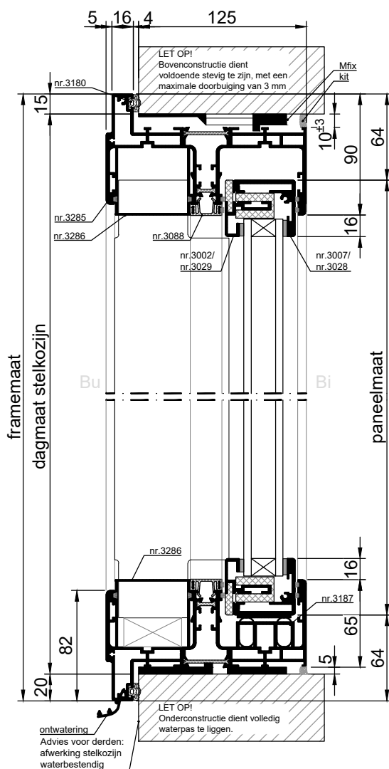
VERTICALE DOORSNEDE type XHS-17A
