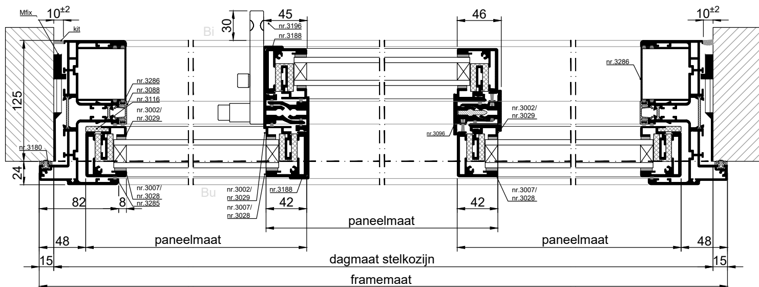
HORIZONTALE DOORSNEDE type XHS-17C
