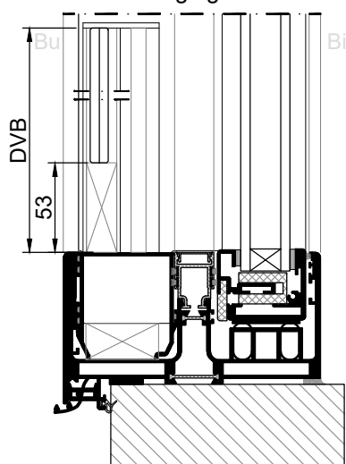
horizontaal onderprofiel met doorvalbeveiliging
