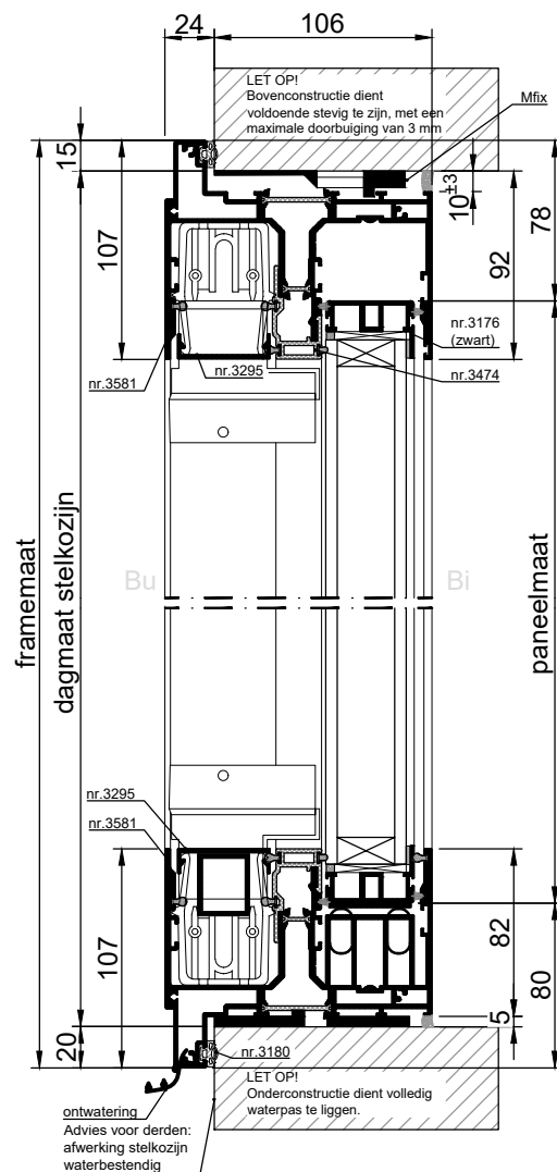
VERTICALE DOORSNEDE type XHS-25E
