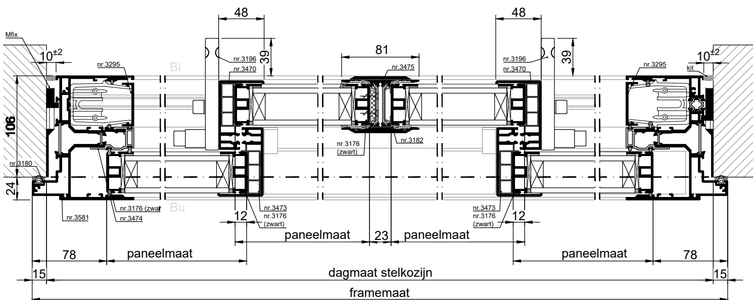
HORIZONTALE DOORSNEDE type XHS-25E
