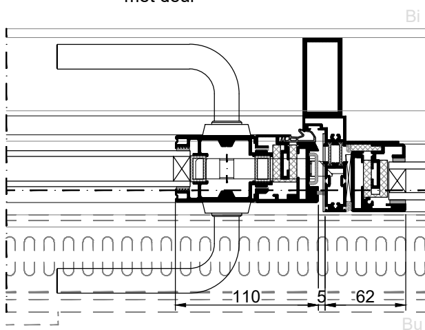
verticale tussenstijl vast paneel met deur
