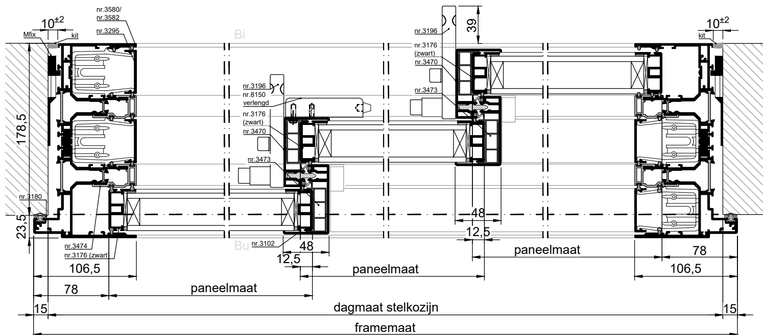
HORIZONTALE DOORSNEDE type XHS-35A
