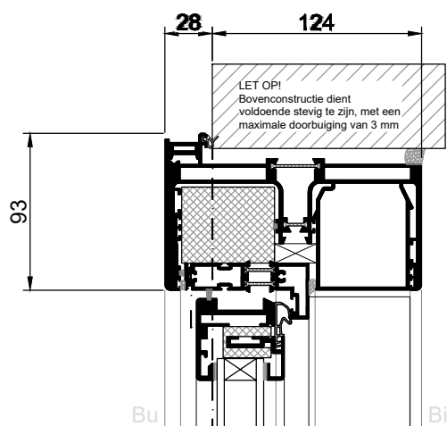
horizontaal bovenprofiel met deur
