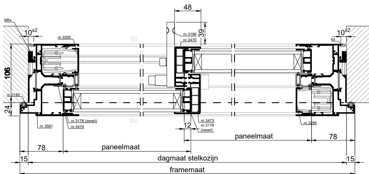
HORIZONTALE DOORSNEDE type XHS-25A
