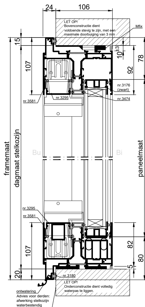
VERTICALE DOORSNEDE type XHS-25A
