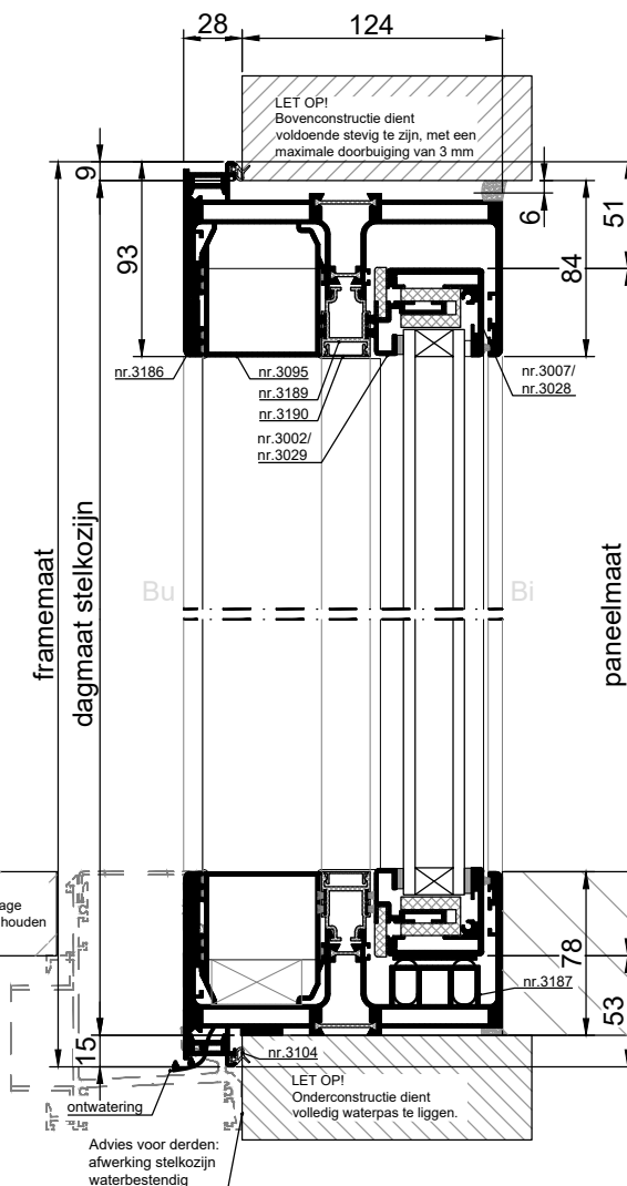
VERTICALE DOORSNEDE type XHS-9E
