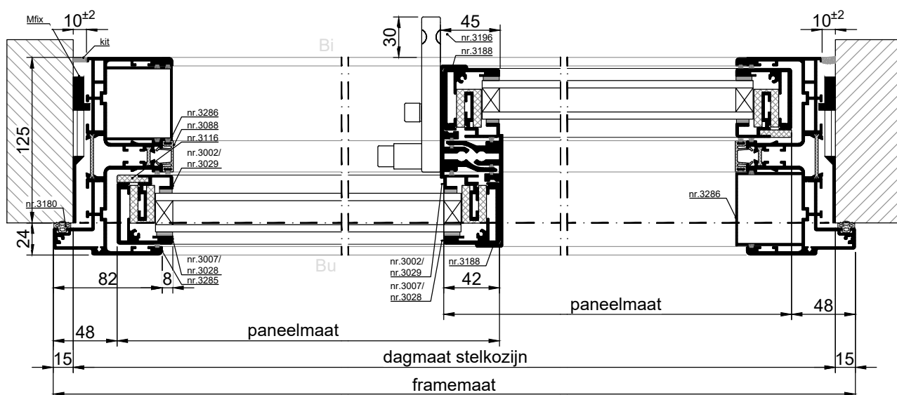
HORIZONTALE DOORSNEDE type XHS-17A
