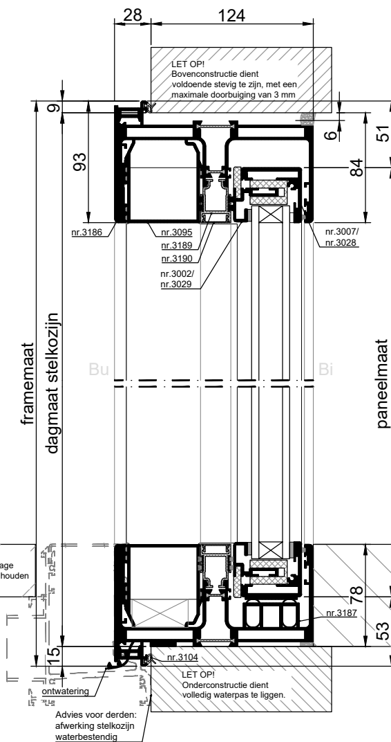
VERTICALE DOORSNEDE type XHS-10E
