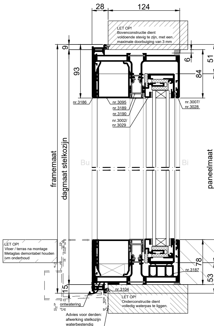
VERTICALE DOORSNEDE type XHS-9C
