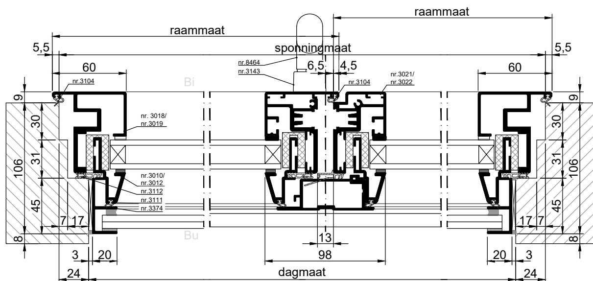
HORIZONTALE DOORSNEDE type MSDK-3
