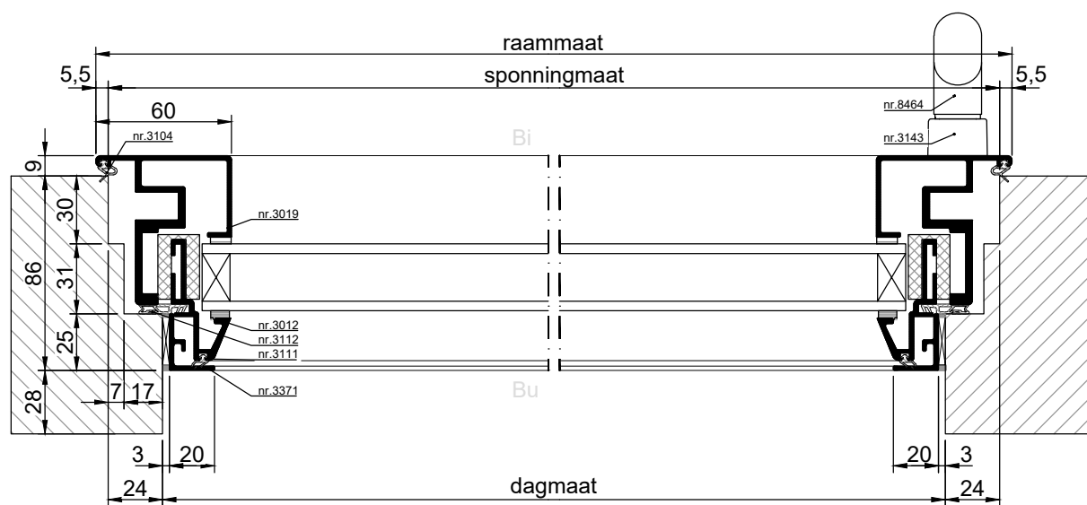
HORIZONTALE DOORSNEDE type MDK-31A
