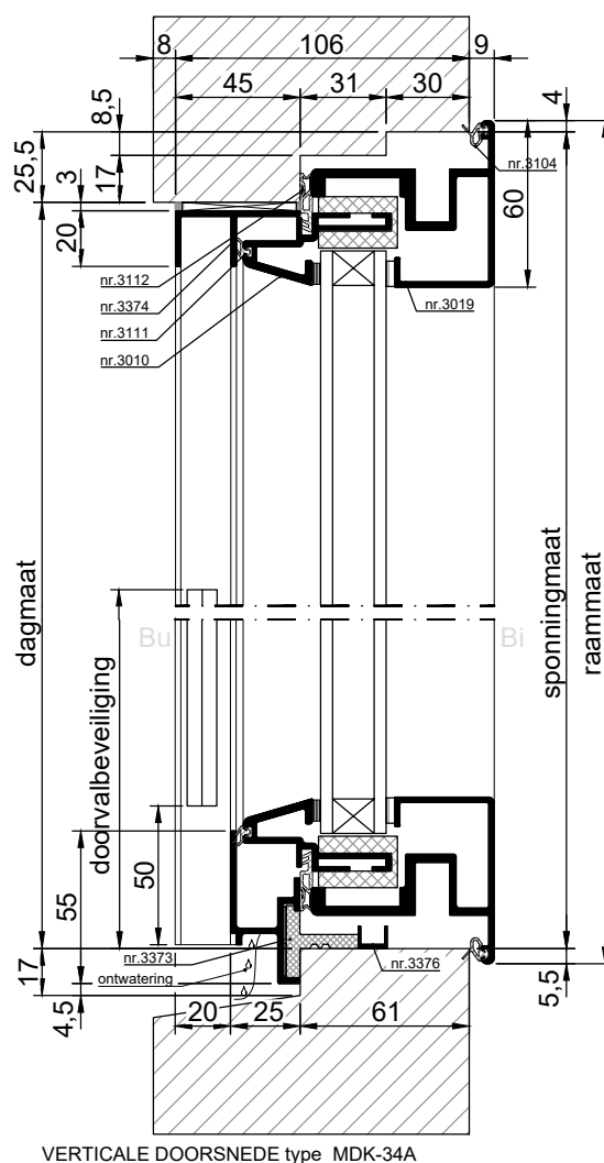
VERTICALE DOORSNEDE type MDK-34A
