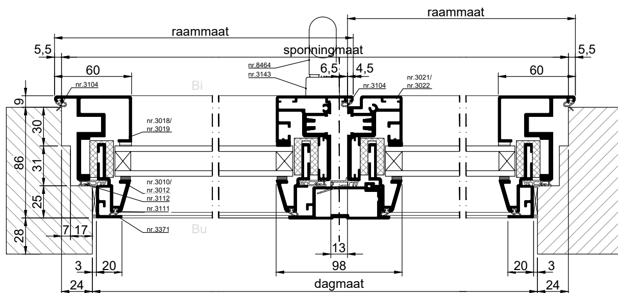
HORIZONTALE DOORSNEDE type MSDK-1
