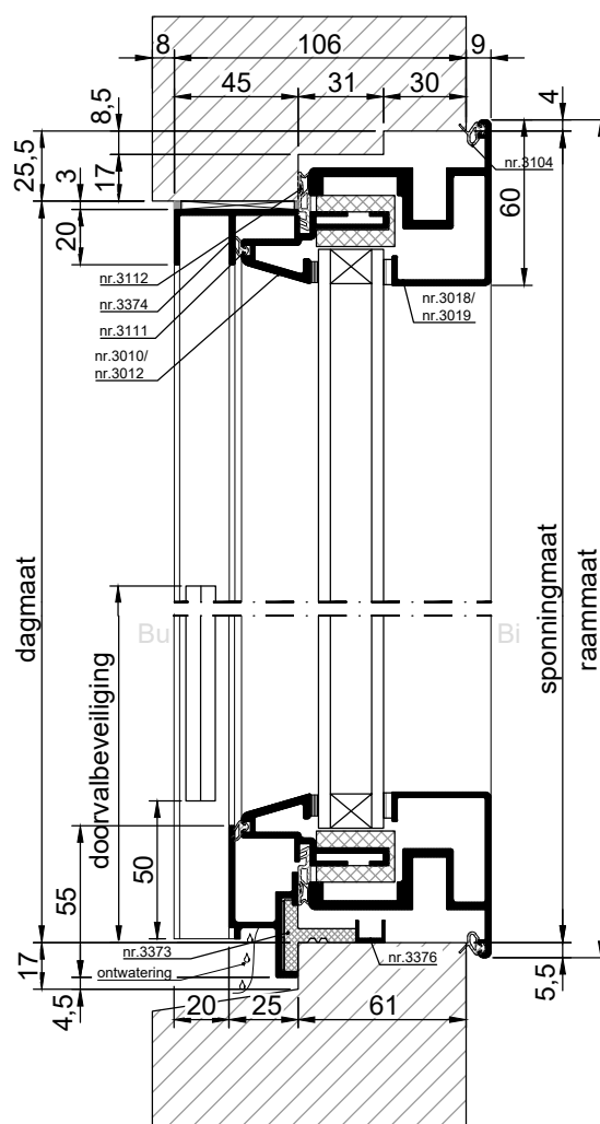
VERTICALE DOORSNEDE type MSDK-3
