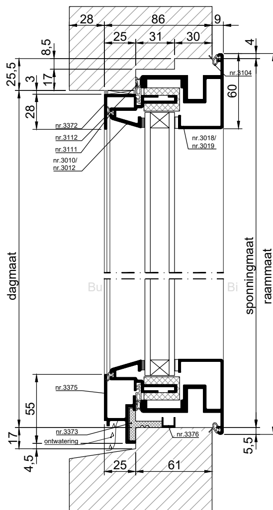
VERTICALE DOORSNEDE type MSDK-1
