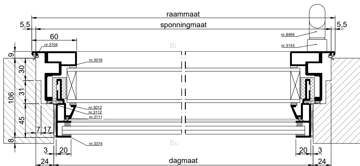
HORIZONTALE DOORSNEDE type MDK-37A
