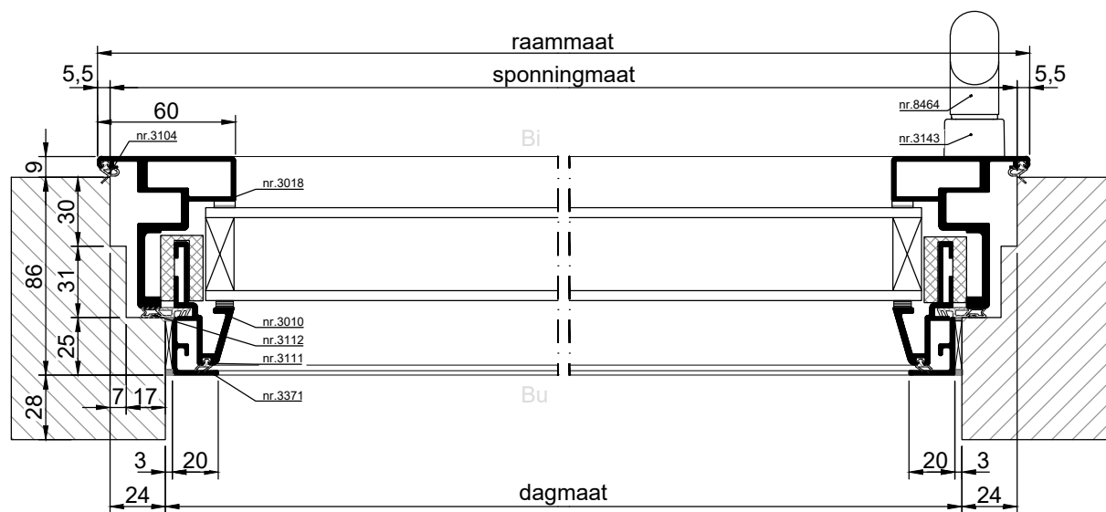
HORIZONTALE DOORSNEDE type MDK-32A
