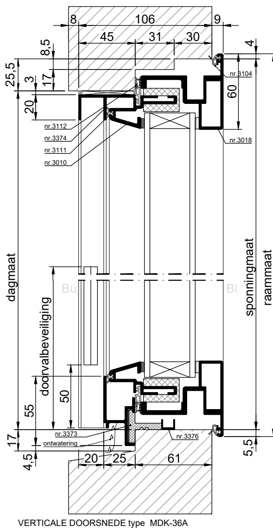
VERTICALE DOORSNEDE type MDK-36A
