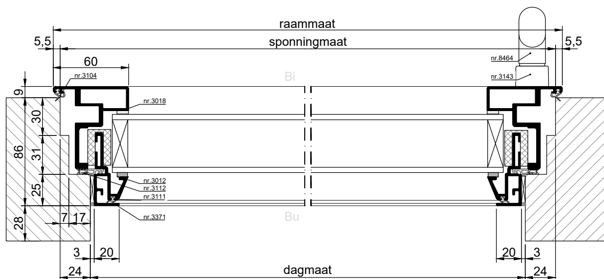
HORIZONTALE DOORSNEDE type MDK-33A
