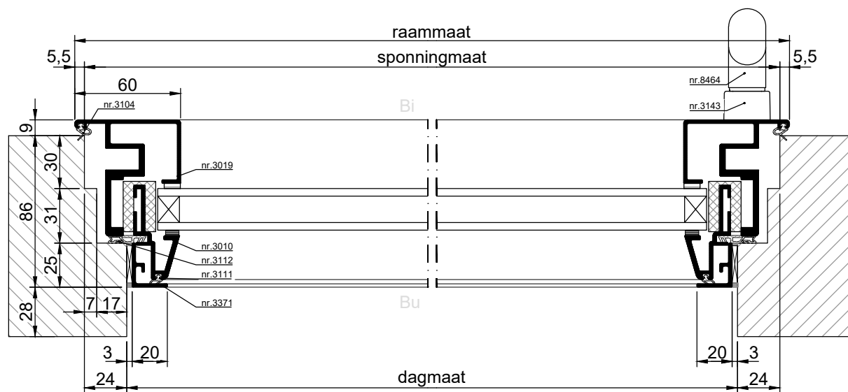
HORizontale DOORSNEDE type MDK-30A
