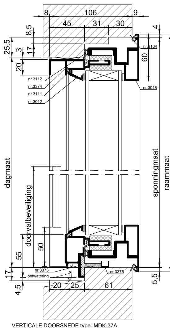
VERTICALE DOORSNEDE type MDK-37A
