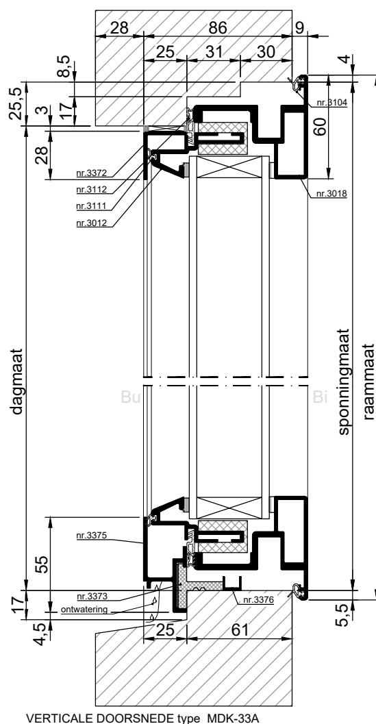
VERTICALE DOORSNEDE type MDK-33A
