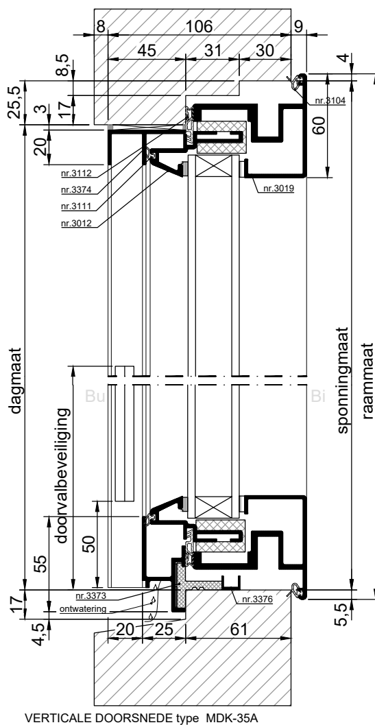
VERTICALE DOORSNEDE type MDK-35A
