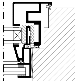
GEÏNTEGREERDE DOORVALBEVEILIGING
