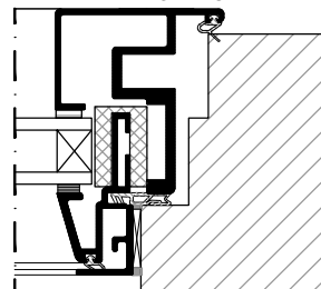
STANDAARD MONTAGE
