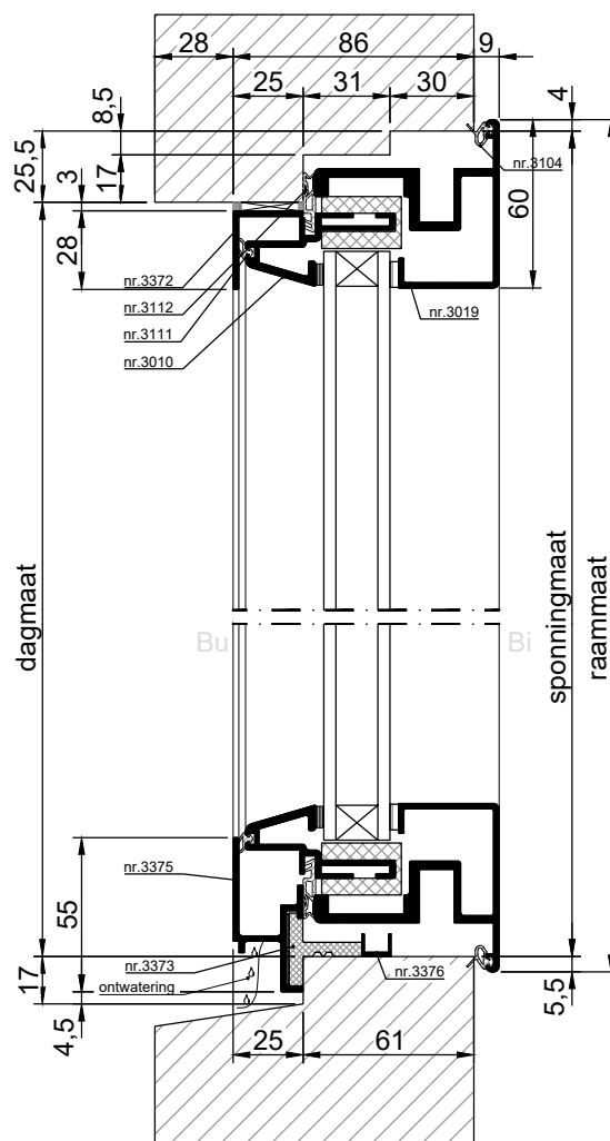
VERTICALE DOORSNEDE type MDK-30A
