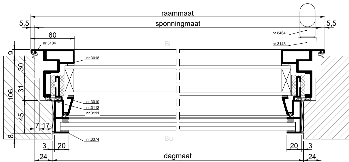
HORIZONTALE DOORSNEDE type MDK-36A
