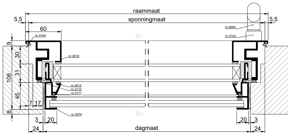
HORIZONTALE DOORSNEDE type MDK-35A
