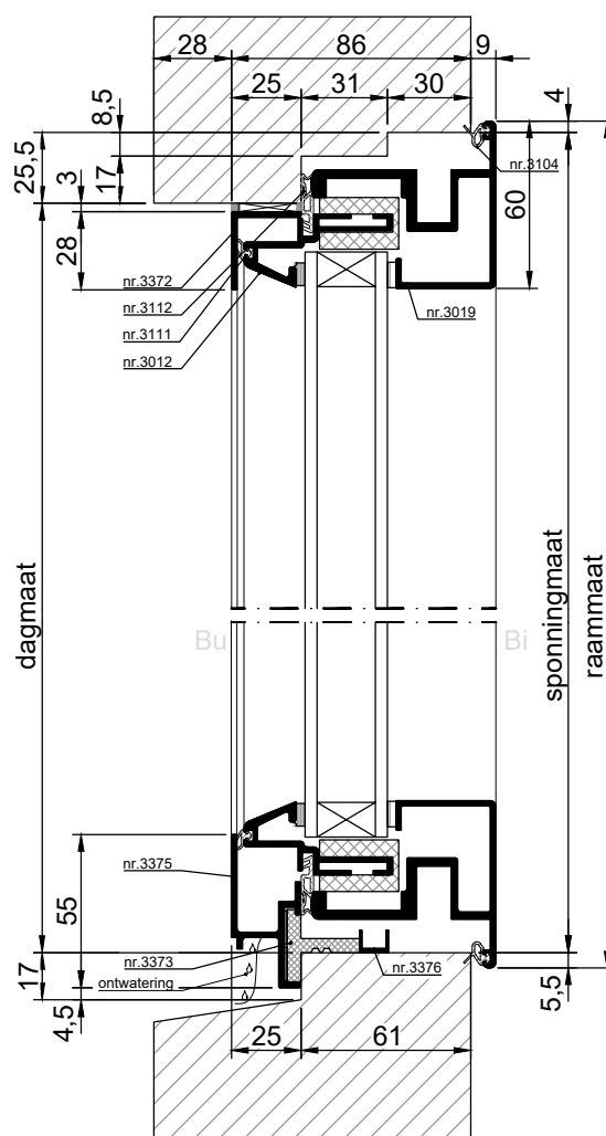
VERTICALE DOORSNEDE type MDK-31A
