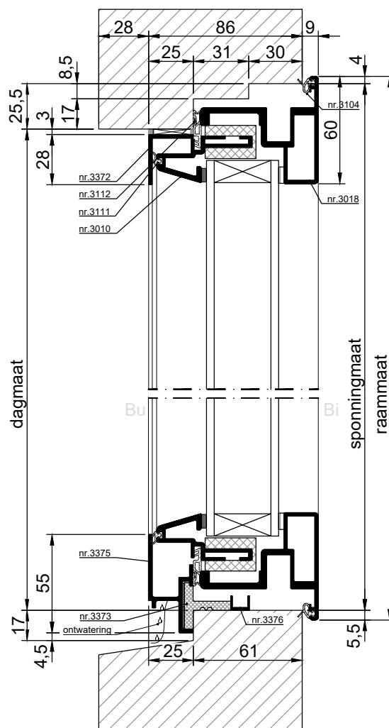
VERTICALE DOORSNEDE type MDK-32A
