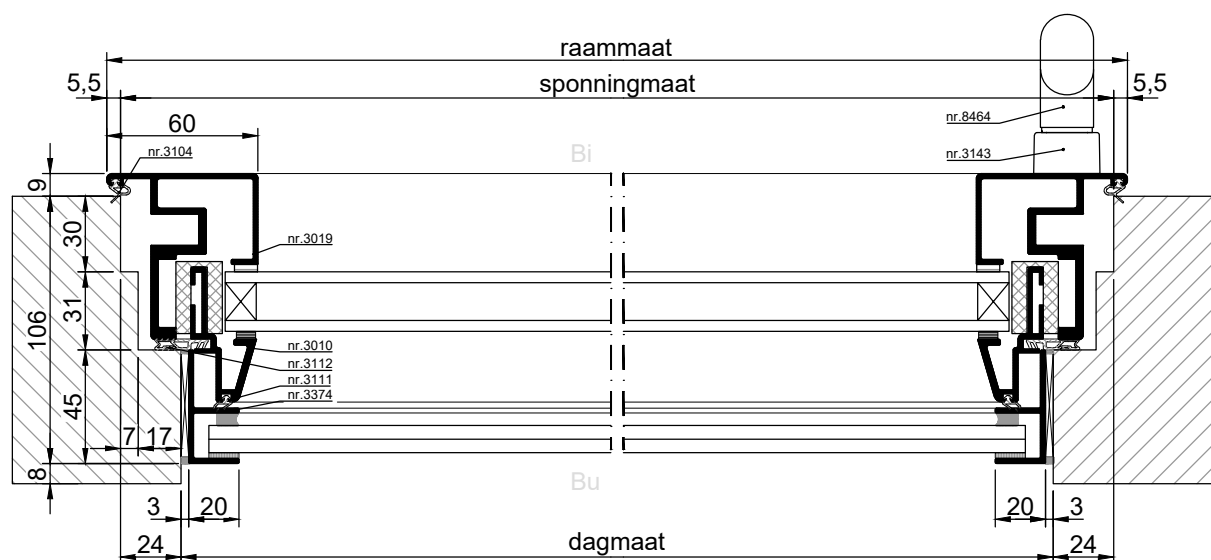
HORizontALE DOORSNEDE type MDK-34A
