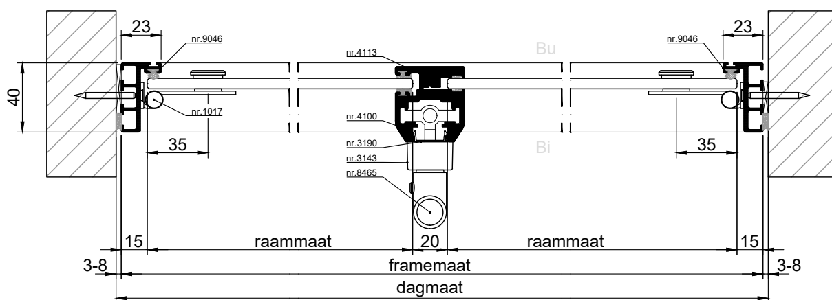
HORIZONTALE DOORSNEDE type SVC-10
