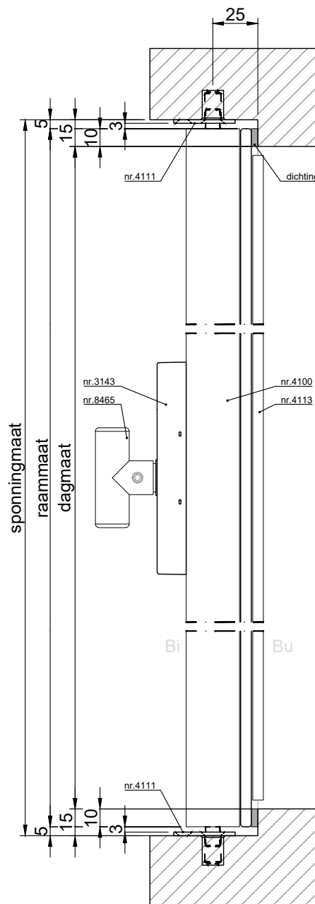
VERTICALE DOORSNEDE type SVR-6
