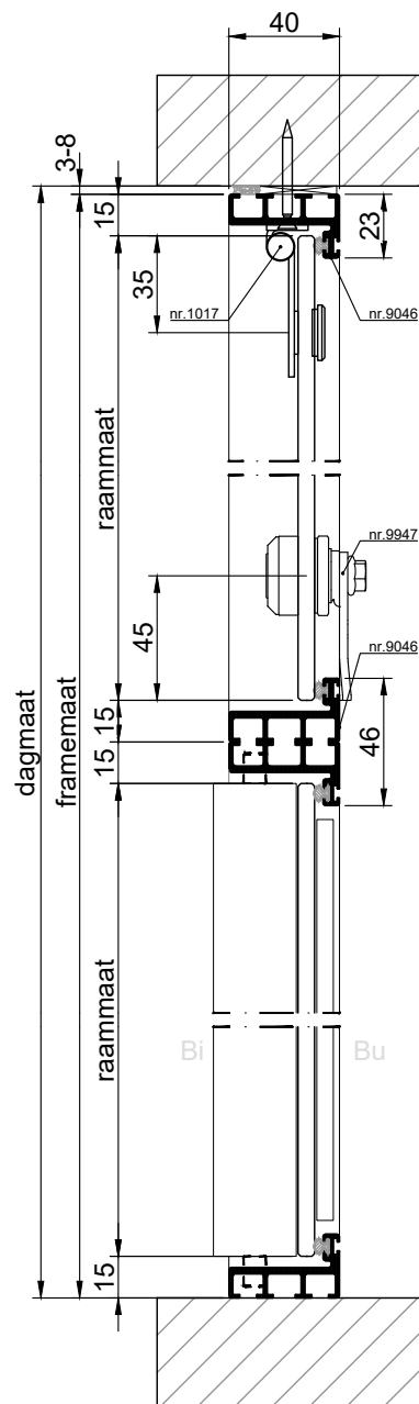
VERTICALE DOORSNEDE type SVC-10
