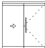
TYPE HSW-2A (zelfsluitend)
