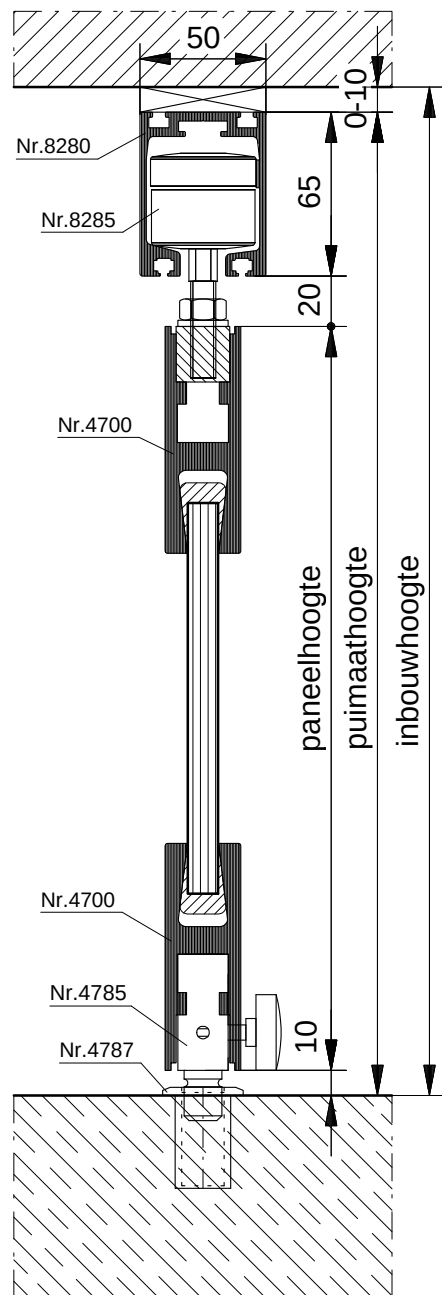
VERTICALE DOORSNEDE HSW-3A
