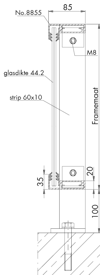
Verticale doorsnede type BW-3
