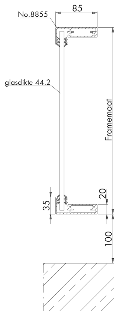
Verticale doorsnede type BW-5
