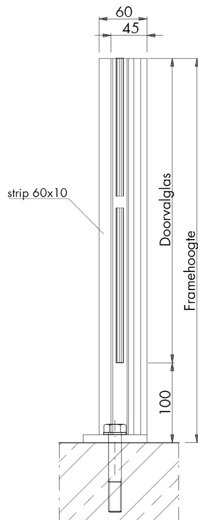
Verticale doorsnede type DVB-1
