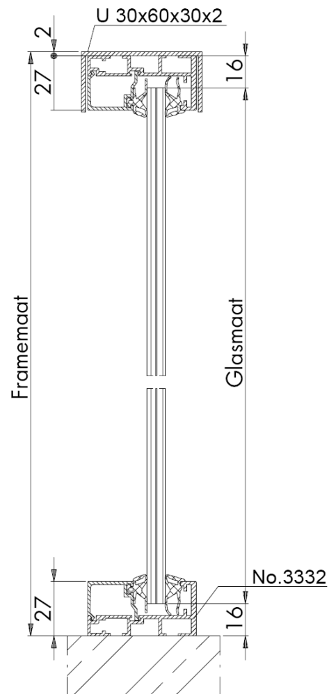
Verticale doorsnede type BW-2
