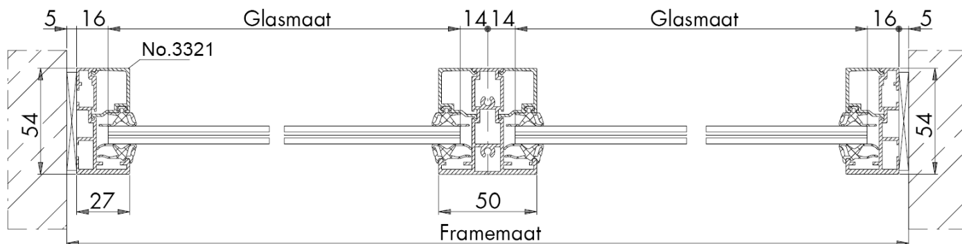
Horizontale doorsnede type BW-2
