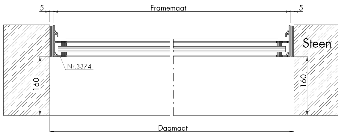
Horizontale doorsnede type DVB-1
