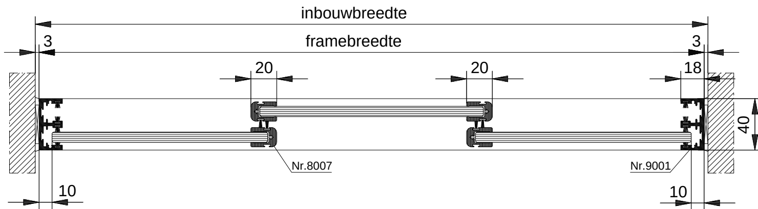
HORIZONTALE DOORSNEDE type ASH-3
