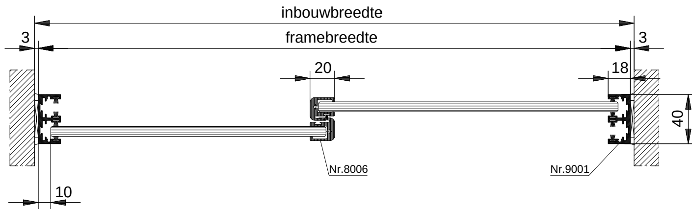
HORIZONTALE DOORSNEDE type ASH-2
