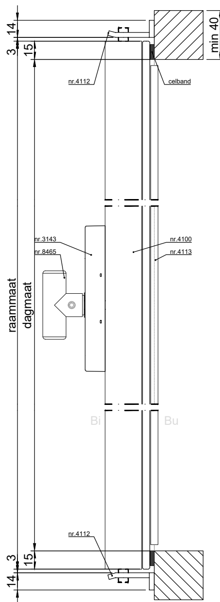
VERTICALE DOORSNEDE type SVR-5
