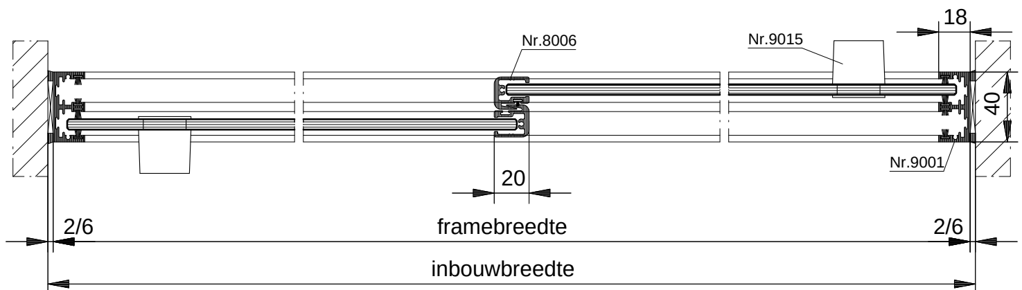
HORIZONTALE DOORSNEDE type HSV-2
